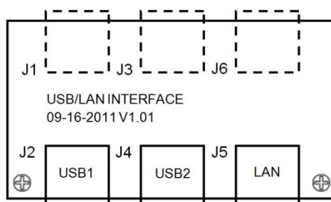
Рисунок 2 – плата USB/LAN INTERFACE
