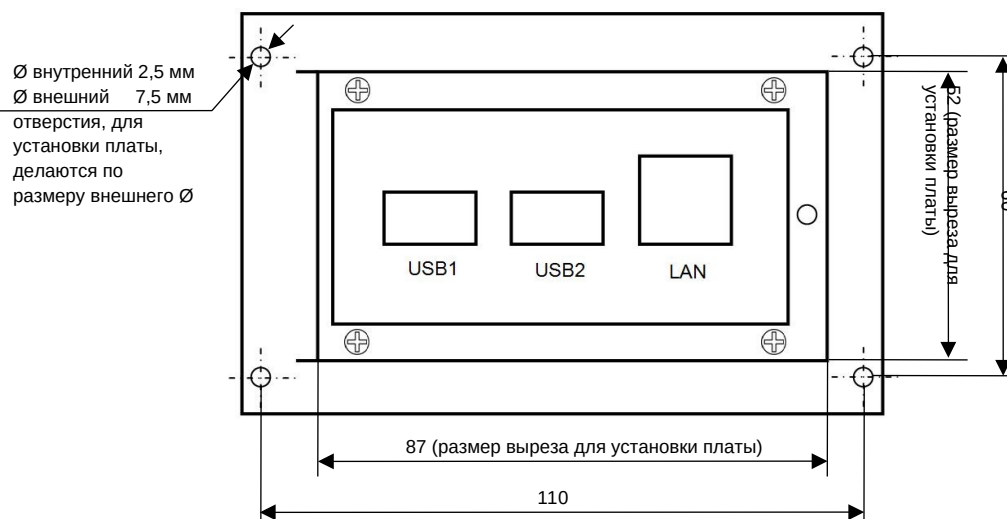
Рисунок 1 – лицевая сторона кросс-платы
